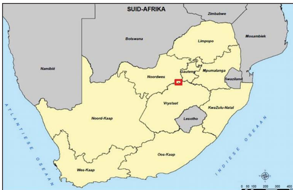
Figuur 1: Oriënteringskaart van die Vredefortkoepel en suidelike Afrika (Landmetergene-raal 2627CB.mxd Okt. 2007)
